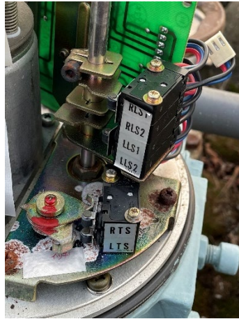
リミットスイッチ交換：東淀川浄水場 排泥促進弁 2 - 8 モーター交換：東淀川浄水場 (手前：新設 奥：既設 (故障))
